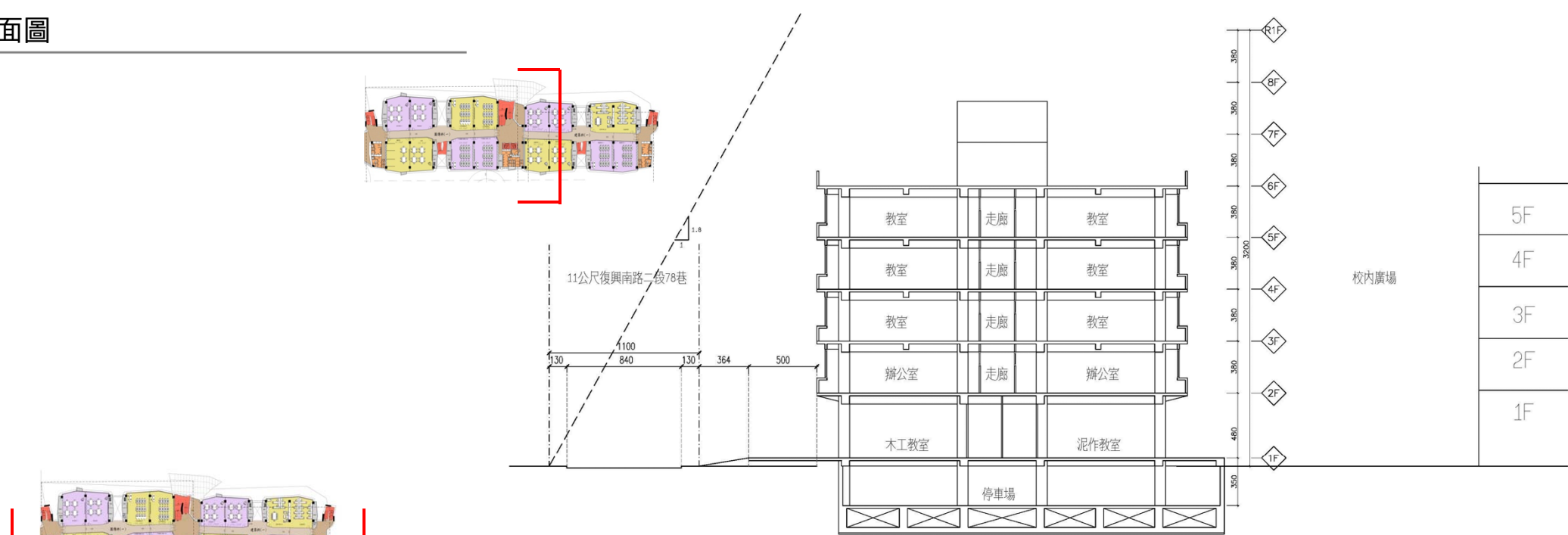
縱向剖面圖 Scale 1/200
