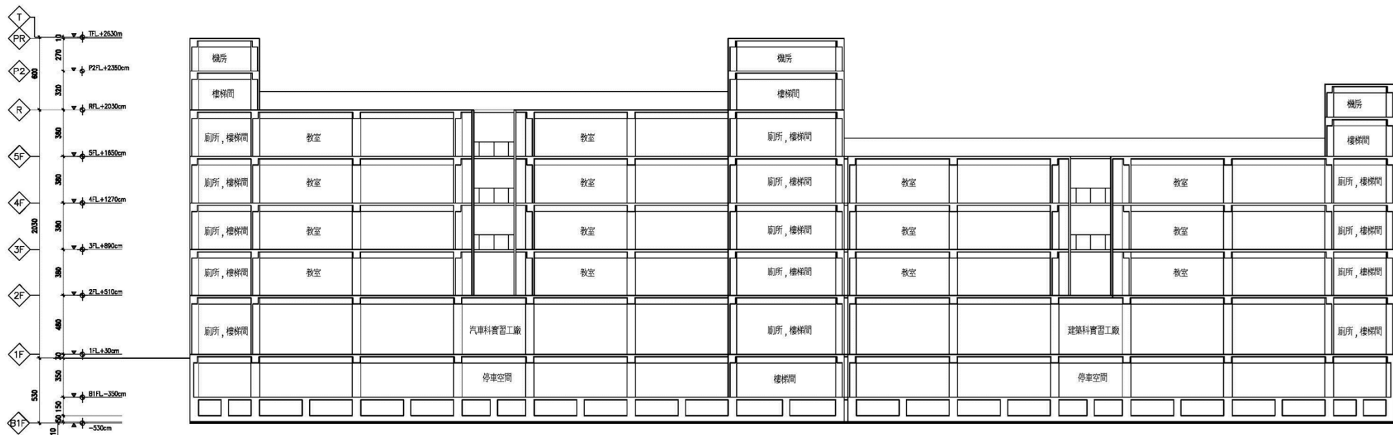
橫向剖面圖 Scale 1/200
